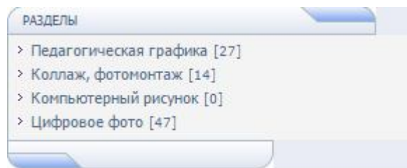
Рис. 6. Выбор раздела
